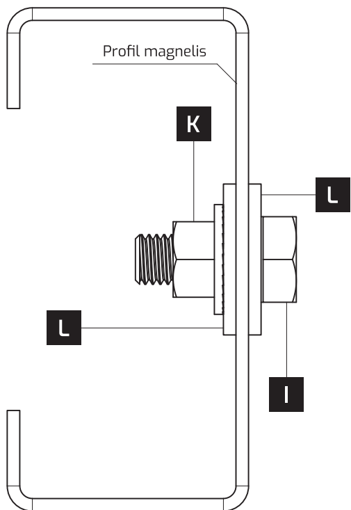
7 Verbindungsmethode für Sechskantschrauben M10
