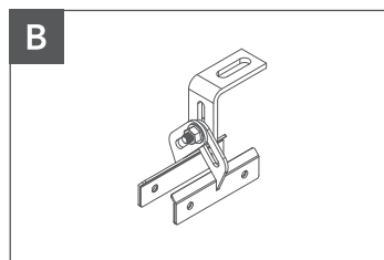
B Uchwyt trapez regulowany DT
