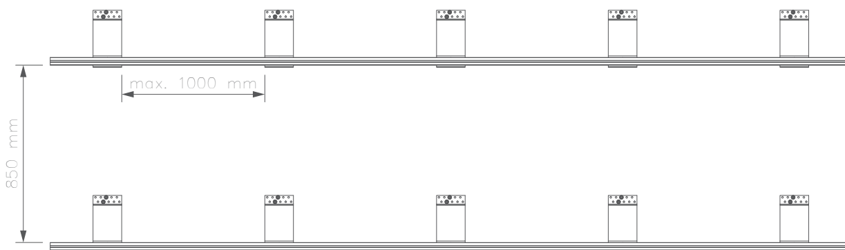
Rys. 2. Rozmieszczenie szyn montażowych wraz z uchwytem dachowym
