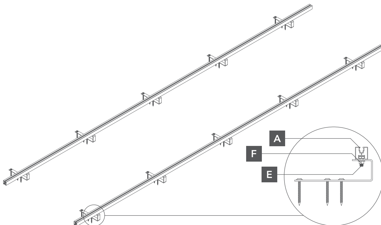
Rys. 6. Mocowanie szyny do uchwyty dachowego
