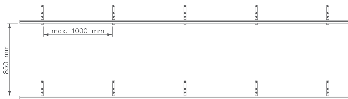
Rys. 2. Rozmieszczenie szyn montażowych wraz z uchwytem dachowym
