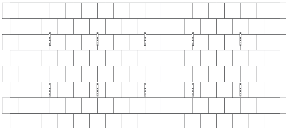
Rys. 3. Wyznaczenie miejsca montażu wsporników konstrukcyjnych
