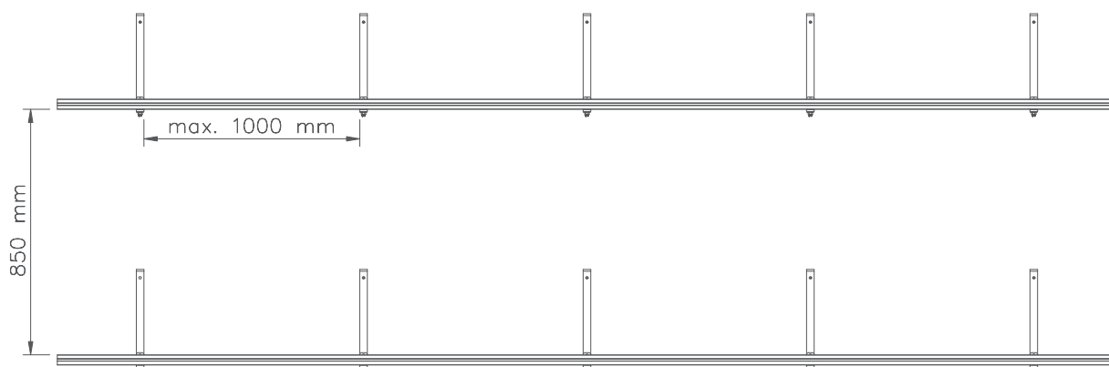
Rys. 2. Rozmieszczenie szyn montażowych wraz z uchwytem dachowym
