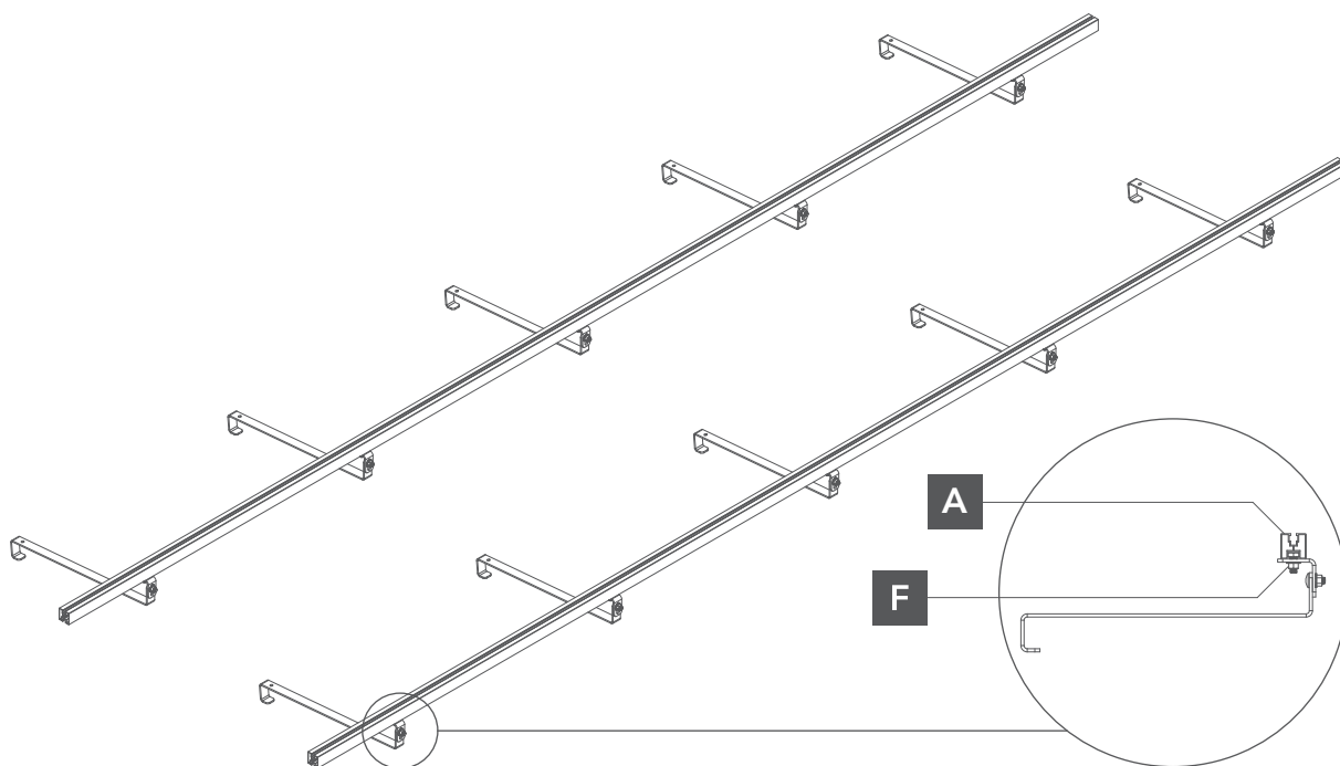
Rys. 6. Mocowanie szyny montażowej do uchwyty dachowego
