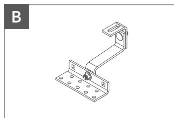
B Uchwyt ceramika regulowany DC1
