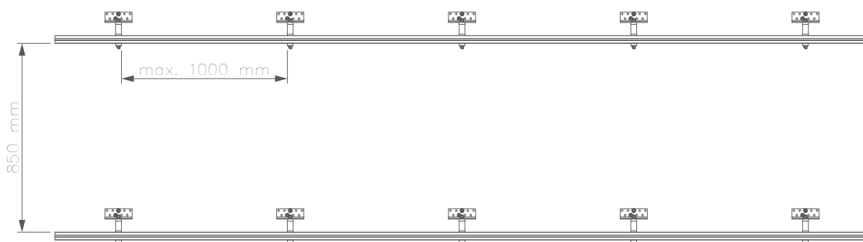
Rys. 2. Rozmieszczenie szyn montażowych wraz z uchwytem dachowym
