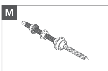
M Śruba z gwintem podwójnym M10
